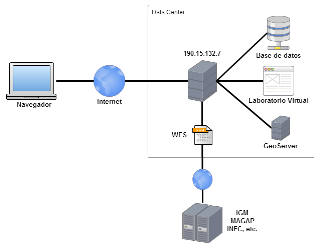
Figura 3. Arquitectura de la plataforma.
